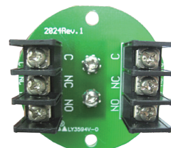
2 SPDT
